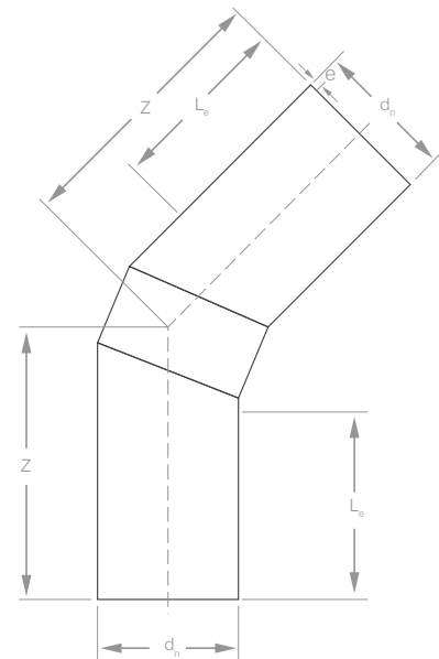
45° Elbow
