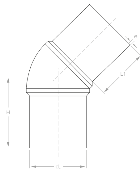
45° Elbow
