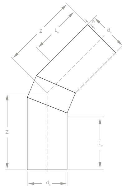
45° Elbow
